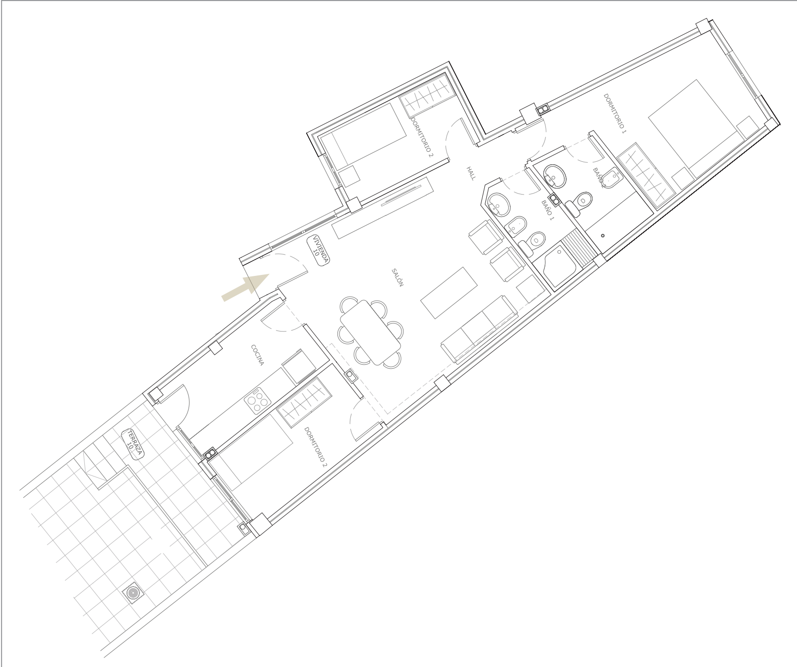
VIVIENDA 10 - 1ª Planta
