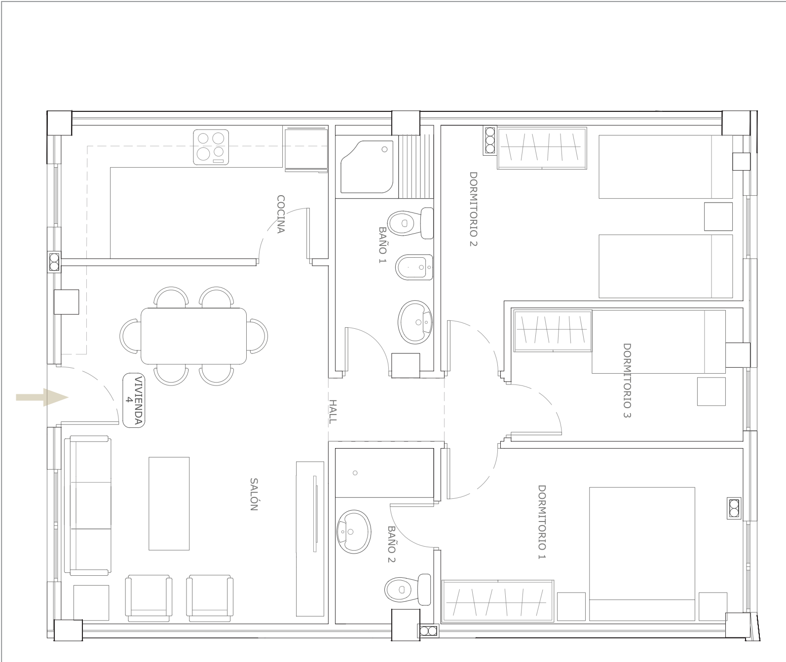
VIVIENDA 4 - Planta Baja
