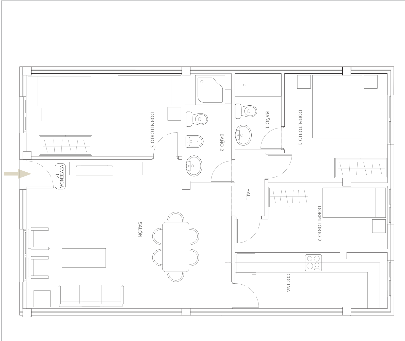
VIVIENDA 14 - 2ª Planta
