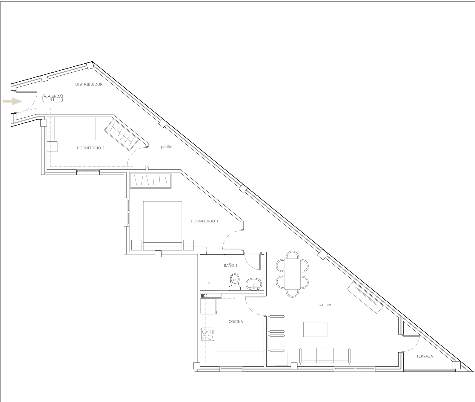
VIVIENDA 41 - Planta Baja
