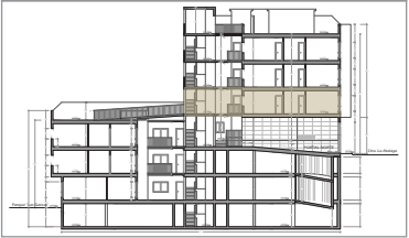
VIVIENDA 10 - 1ª Planta
