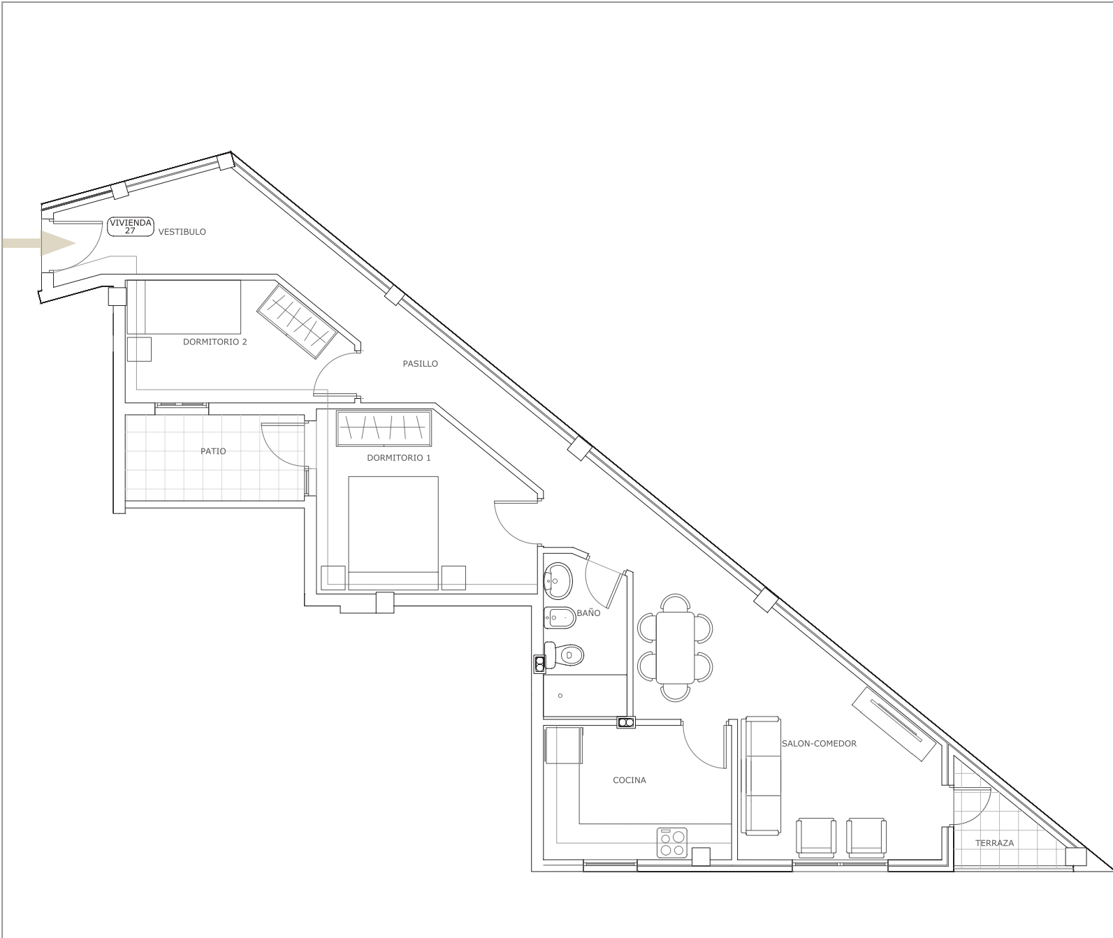
VIVIENDA 27 - Planta Baja Sur
