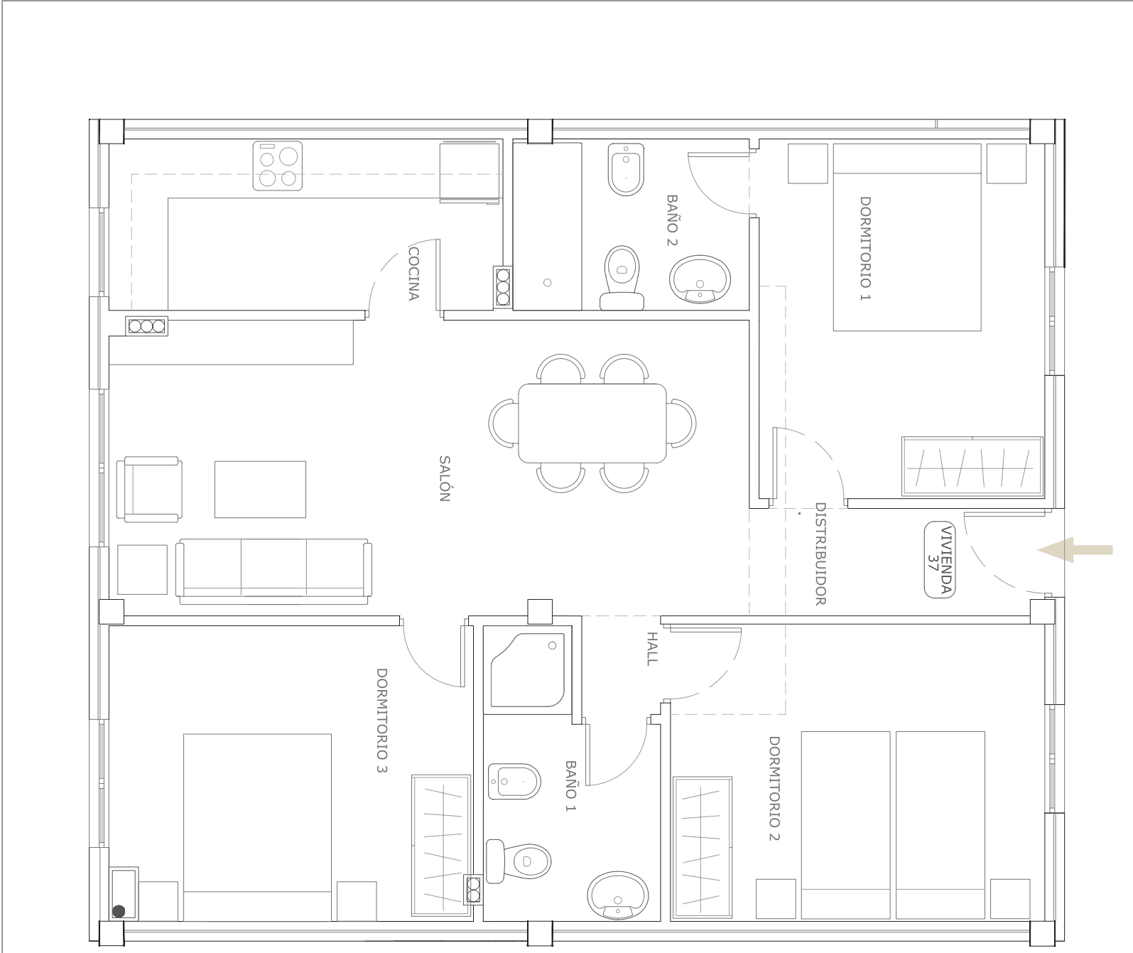
VIVIENDA 37 - Planta Baja
