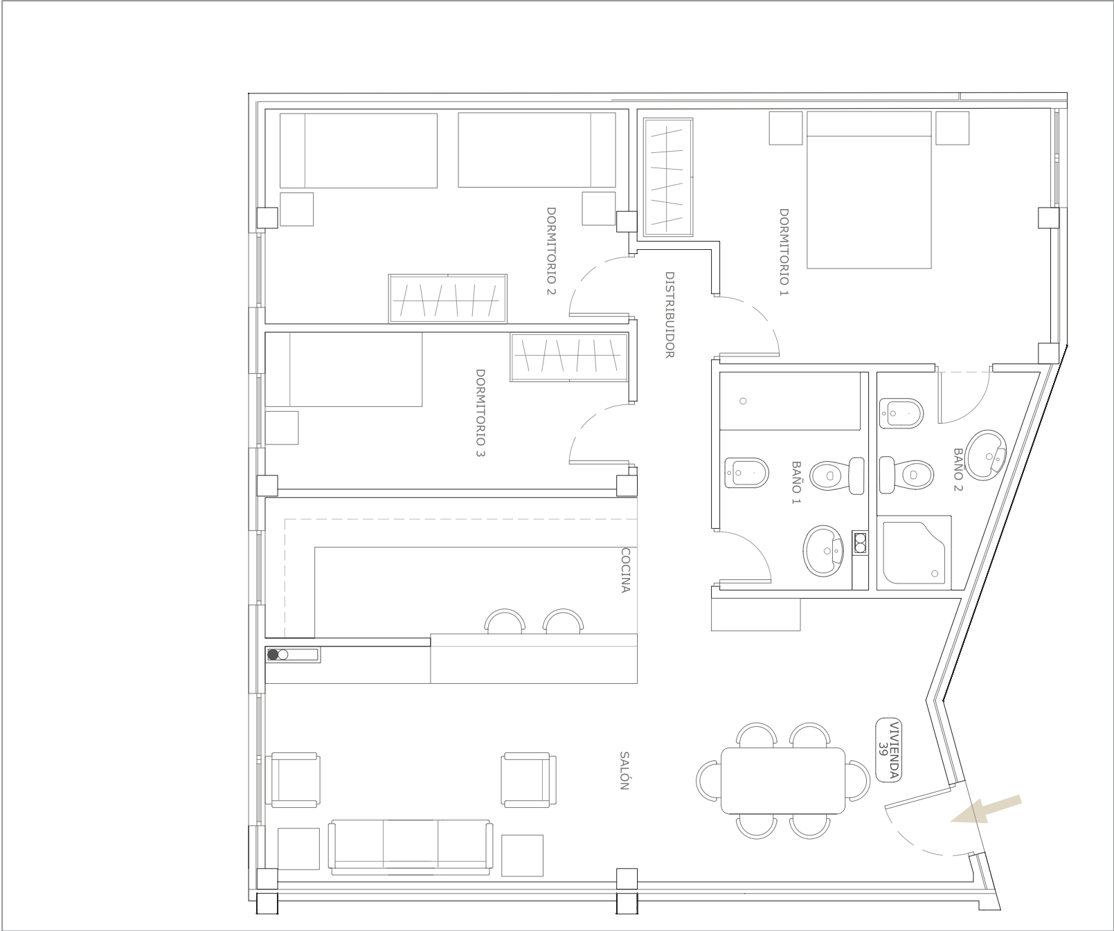
VIVIENDA 39 - Planta Baja
