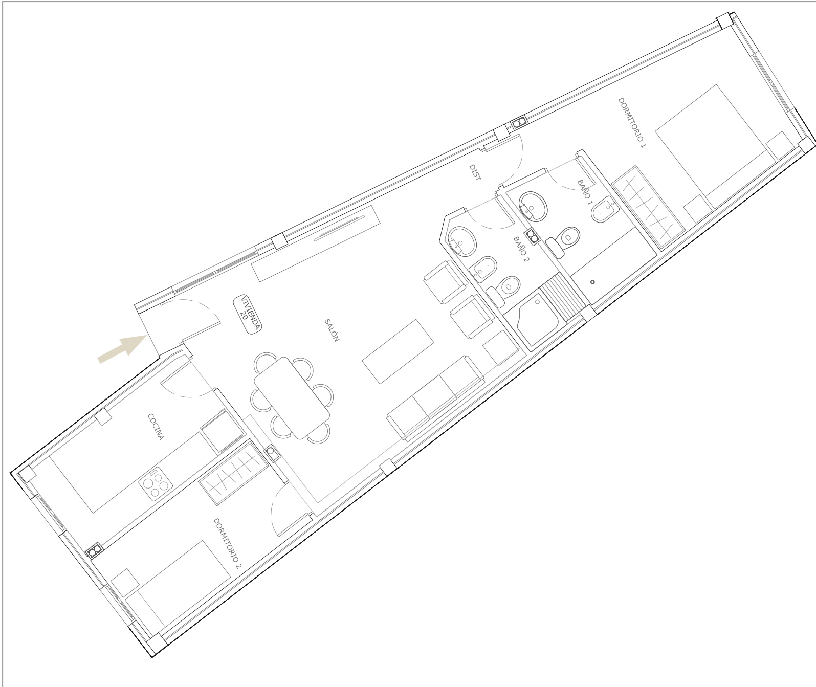
VIVIENDA 20 - 3ª Planta
