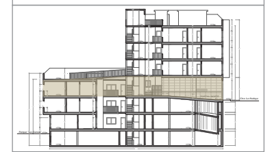
VIVIENDA 36 - Planta Baja
