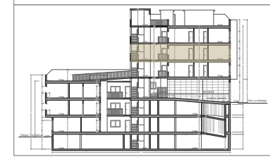
VIVIENDA 14 - 2ª Planta
