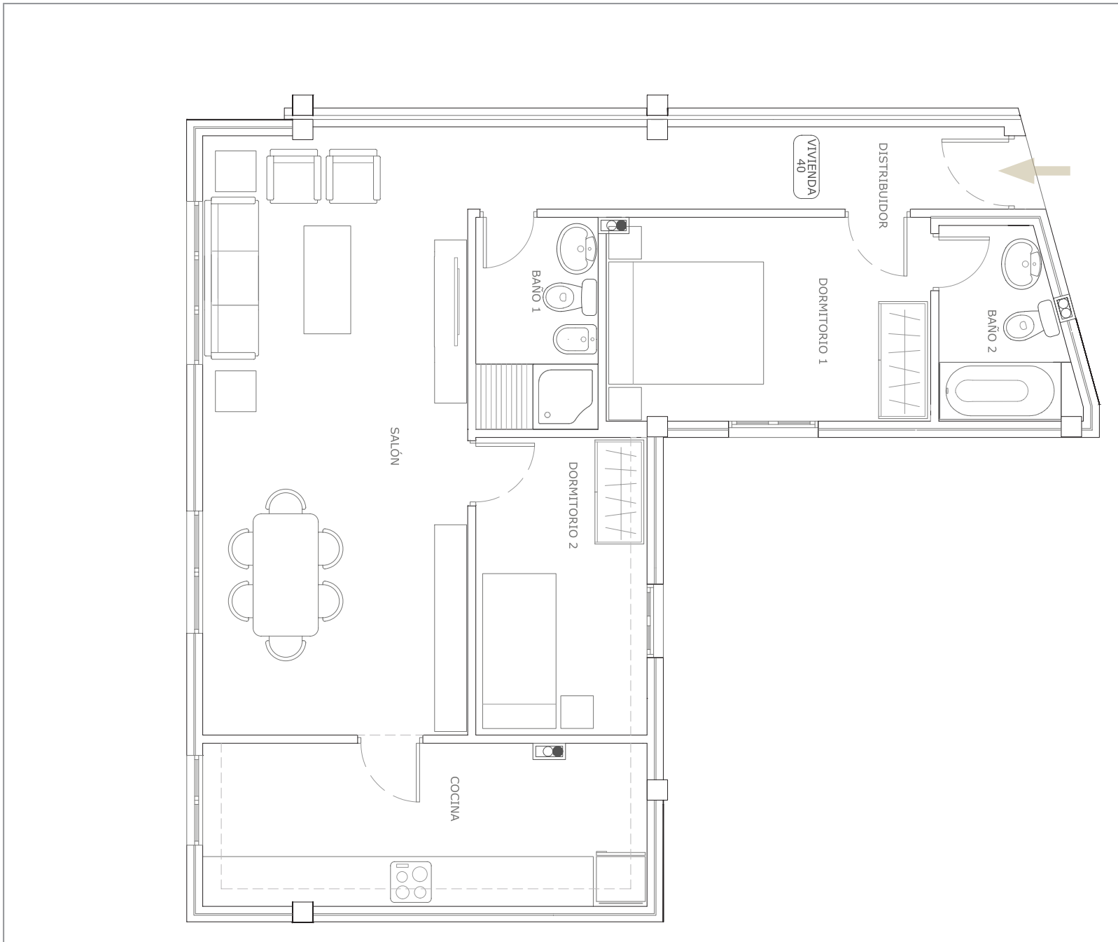
VIVIENDA 40 - Planta Baja
